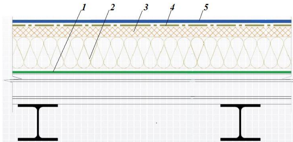
Рисунок 3. Система неэксплуатируемой крыши по стальному профилированному настилу: 1 — пленка пароизоляционная; 2 — минераловатный утеплитель; 3 — плиты теплоизоляционные PIR; 4 — стеклохолст; 5 — полимерная мембрана
