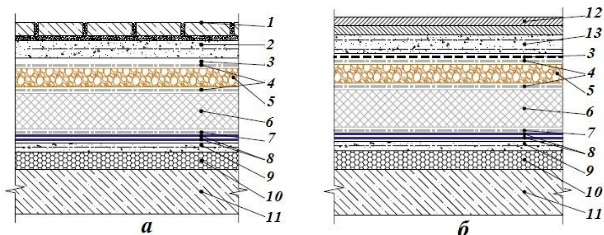
Рисунок 1. Схема эксплуатируемой крыши: а — под пешеходную нагрузку; б — под транспортную нагрузку;
